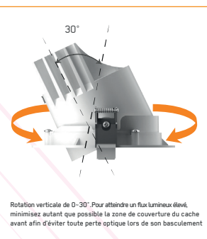
Luminaires Directionnel
