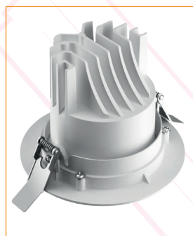
Rotation verticale de 0-30°. Pour atteindre un flux lumineux élevé, minimisez autant que possible la zone de couverture du cache avant afin d'éviter toute perte optique lors de son basculement
